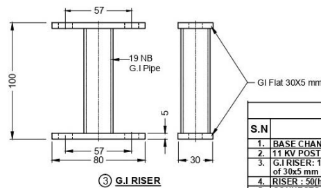
③ G.I RISER
