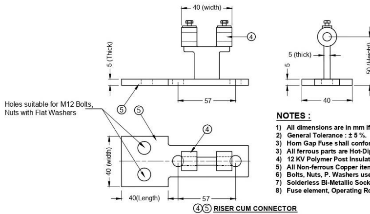
④⑤ RISER CUM CONNECTOR
